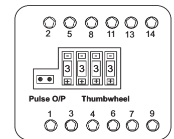
Rear View of RISH EM 3490
