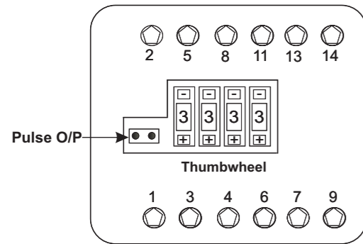
Rear View of RISH EM 3490
