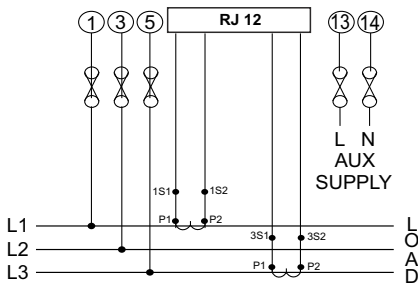
b) 3 Phase 3 Wire
