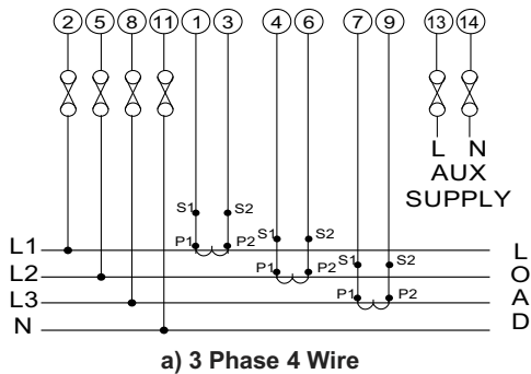
a) 3 Phase 4 Wire
