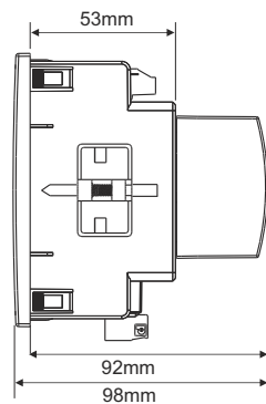
c) Ethernet + 2DI + 2DO
